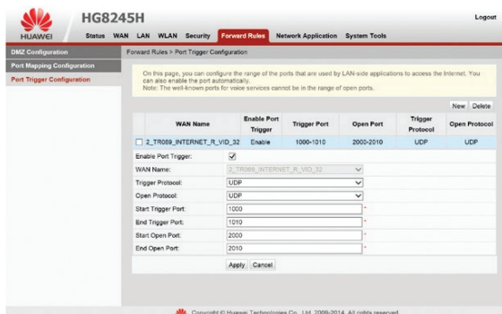
6.24. ábra: Port Trigger beállítás
