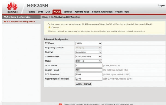
6.17. ábra: WiFi kapcsolat haladó szintű beállításai
