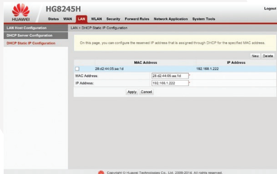
6.15. ábra: DHCP statikus IP cím beállítása
