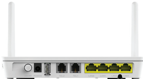
5.1. ábra: A készülék csatlakoztatása (hátlap)
